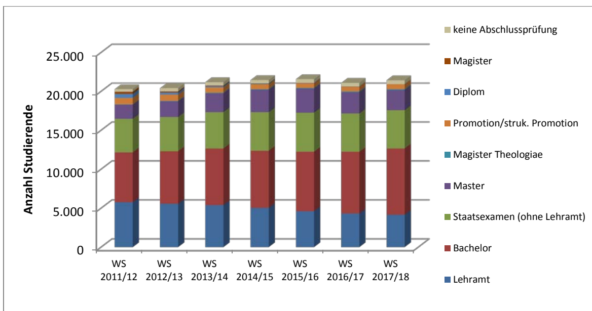
Abbildung 5: Entwicklung der Studierendenzahlen nach Studienzielen von Wintersemester 2011/12 bis Wintersemester 2017/18
