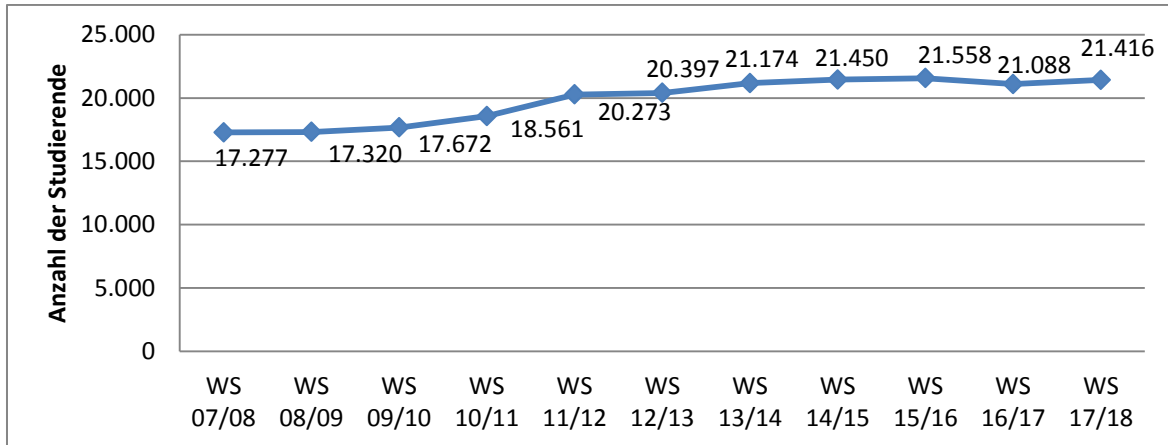
Abbildung 4: Entwicklung der Anzahl der Studierenden an der Universität Regensburg seit Wintersemester 2006/07
