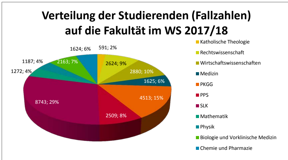
Abbildung 6: Verteilung der Studierenden (Fallzahlen) auf die Fakultät an der Universität Regensburg im Wintersemester 2017/18
