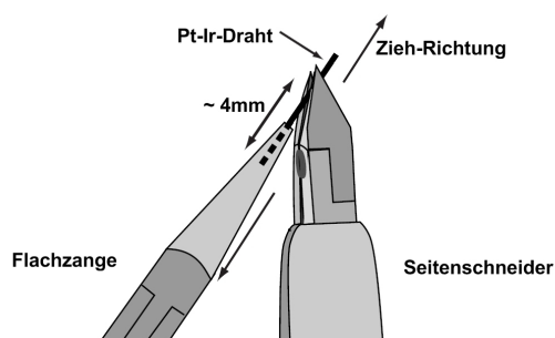
Abbildung 2.8: Schneiden eines Pt-Ir-Drahtes, Abb. aus [1].
