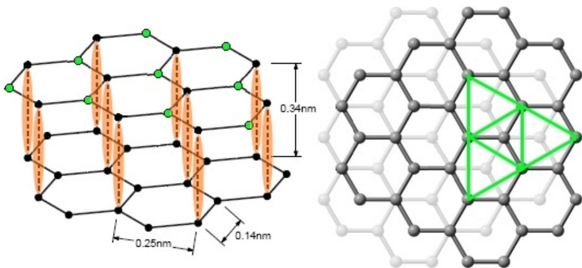
Abbildung 2.11: links: Kristallstruktur von Graphit, rechts: Draufsicht. Abb. aus [1].
