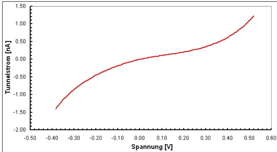
Abbildung 4.22: nichtlineare Strom-Spannungs-Kennlinie
