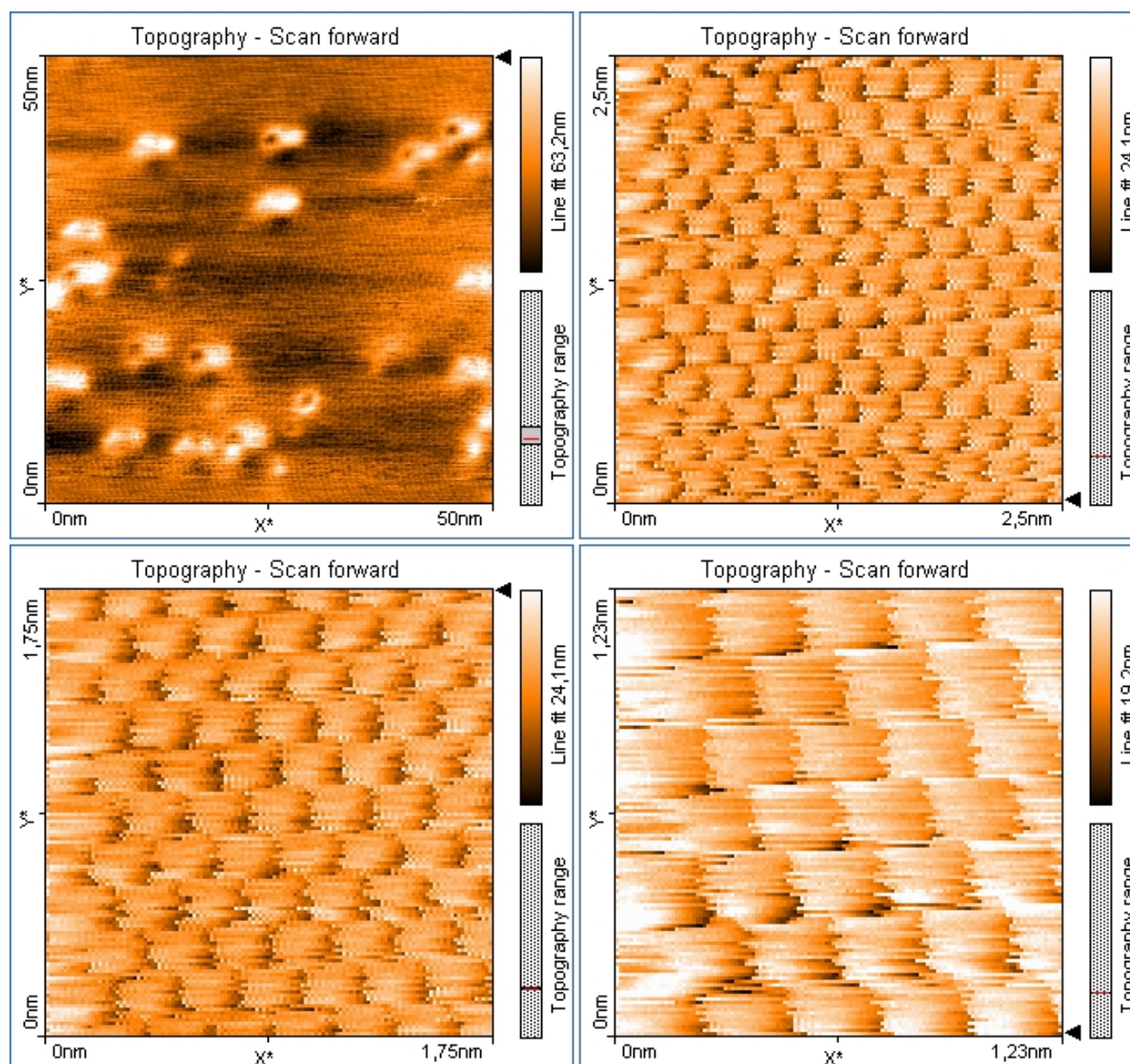
Abbildung 4.21: Die MoS 2 Probe in verschiedenen Auflösungsbereichen
