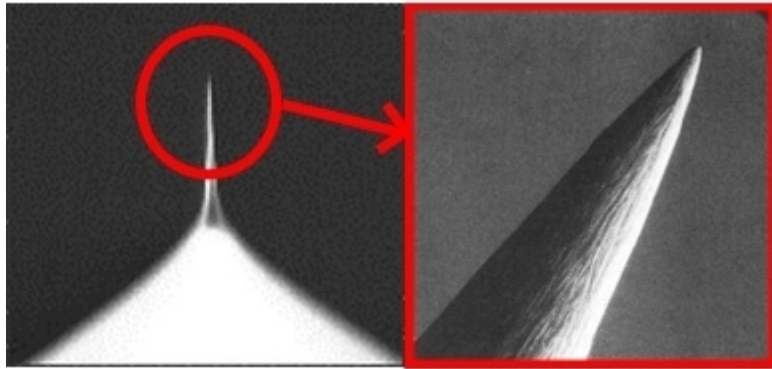
Abbildung 2.9: Durch elektrochem. Ätzen hergestellte Wolframspitze, Abb. aus [12].
