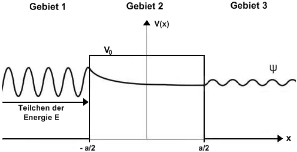
Abbildung 2.2: Eindimensionaler Tunneleffekt
