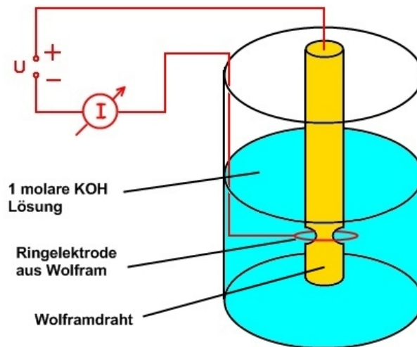
Abbildung 2.10: Aufbau einer Vorrichtung zum elektrochemischen Ätzen von Spitzen.
