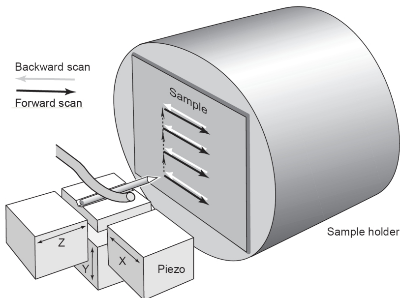
Abbildung 2.6: Die Piezoelemente rastern die Spitze über die Oberfläche. Abb. aus [1].
