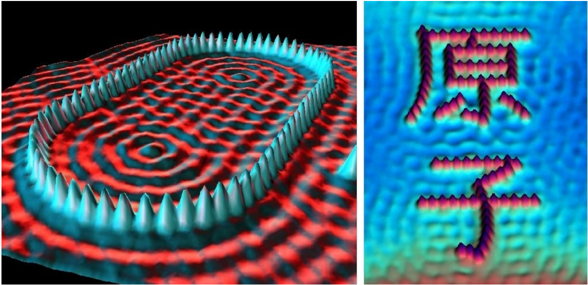
Abbildung 1.7: links: Quantentrog, Eisenatome auf Kupfer (111) rechts: Atom, Eisenatome auf Kupfer (111) Abb. aus [18].
