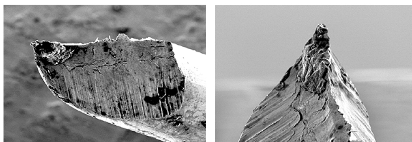
Abbildung 2.7: Pt-Ir-Spitze, Abb. aus [1].
