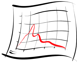
Abbildung 2: Enterprise Model
